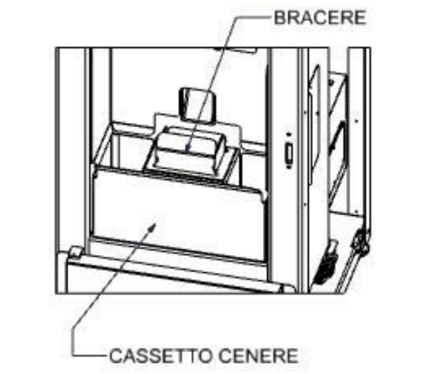
Figura 7 Camera di combustione.
