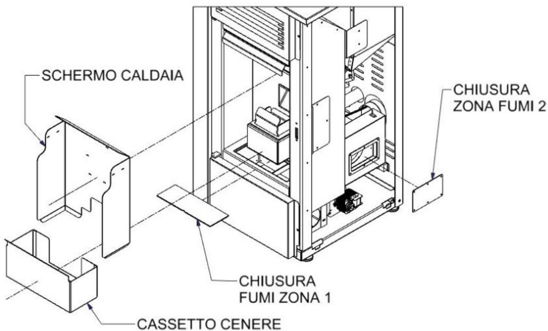
Figura 8 Caldaia completa e Caldaia con particolari rimossi per pulizia
